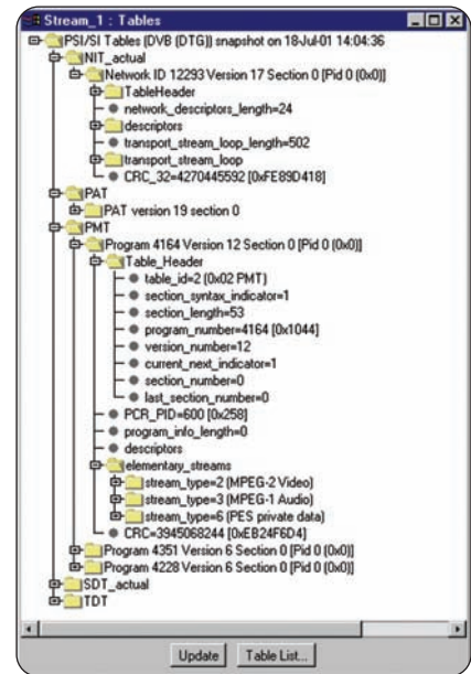
▶ MTM400 SI tables.
